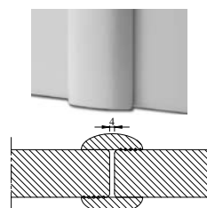
AC9203 AANSLAGLAT ROND
