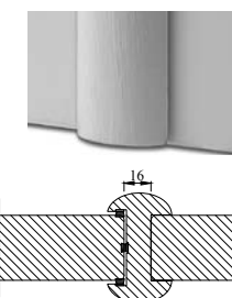
AC9253 SCHUIFDEURNAALD SOFT-STOP ROND
