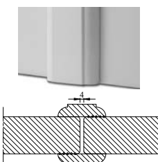
AC9202 AANSLAGLAT KRAAL
