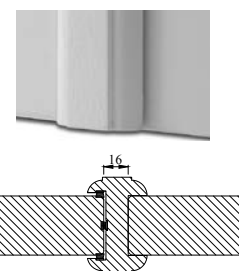
AC9252 SCHUIFDEURNAALD SOFT-STOP KRAAL
