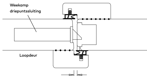
Dubbele deursluiting 3 (binnendraaiend)
