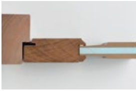
Doorsnede geïsoleerde deur 54 mm.
